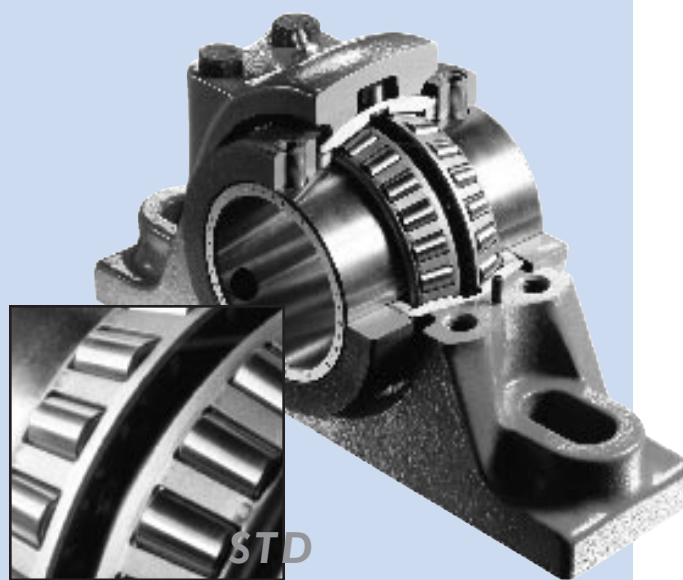
Metal Cage
